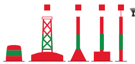
Backbordseite des durchgehenden Fahrwassers/Steuerbordseite des abzweigenden oder einmündenden Fahrwassers
